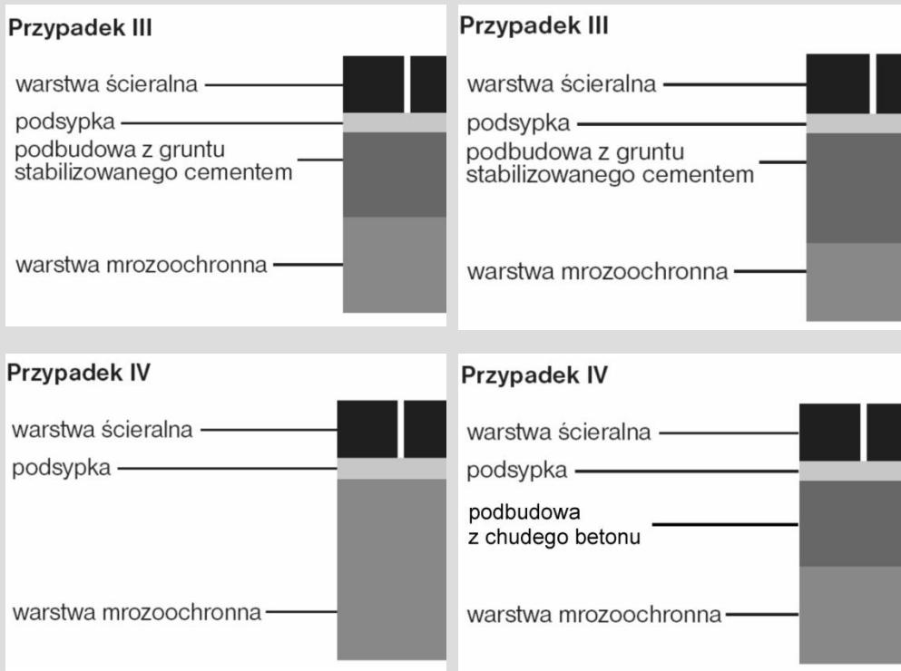
2.3. Konstrukcja nawierzchni dla kategorii ruchu R_2 – grubość warstwy w [cm]
