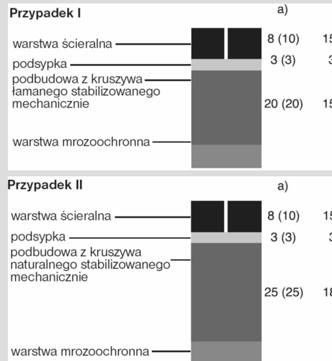
2.4. Konstrukcja nawierzchni dla kategorii ruchu R_3 – grubość warstwy w [cm]
