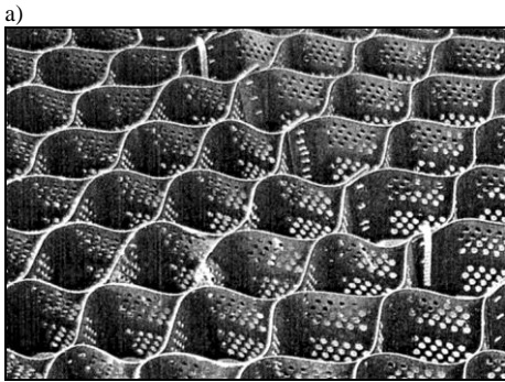
Rys. 7. Ułożona i wypełniona geosiatka komórkowa a) Geosiatka po ułożeniu, b) Geosiatka przymocowana do podłoża kotwami i częściowo zasypana, c) Geosiatka całkowicie zasypana kruszywem
