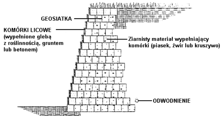
c) Przekrój poprzeczny ściany oporowej z geosiatki komórkowej z licem ściany lekko pochylonym
