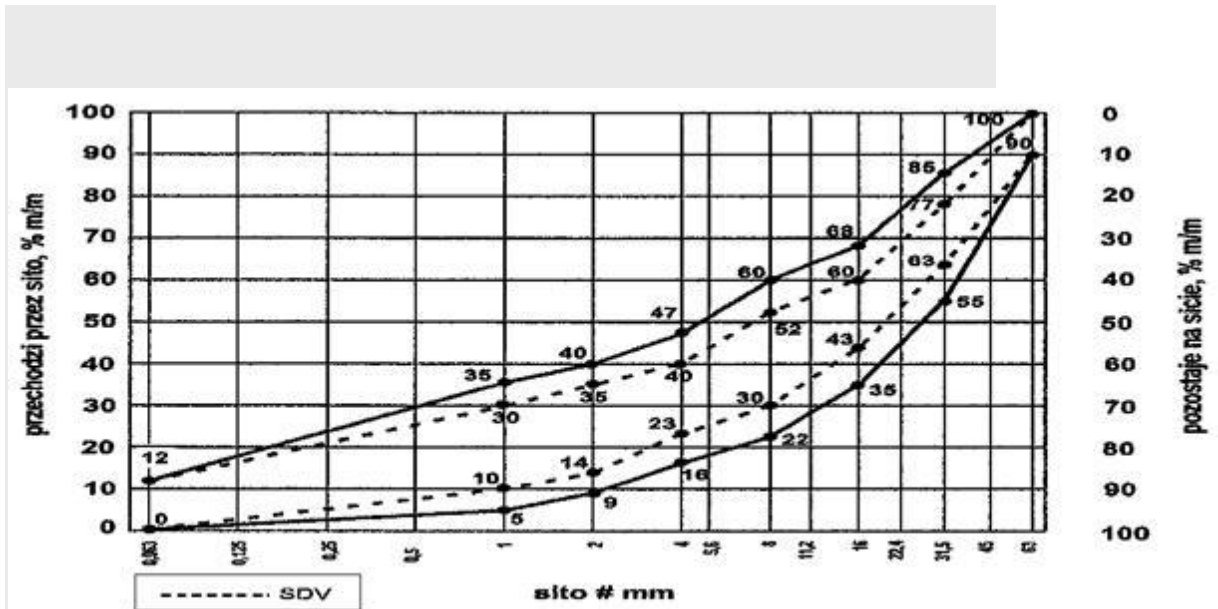
Rys. 3. Krzywe graniczne uziarnienia mieszanki kruszywa niezwiązanego 0/63 mm do warstw podbudowy pomocniczej
