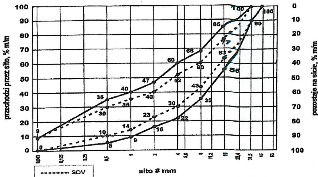
Rysunek 1. Uziarnienie mieszanki niezwiązanej 0/31,5 do podbudowy
